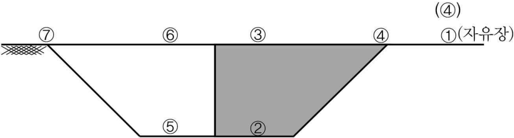
[별도 11] 필댐과 콘크리트댐의 합성댐인 경우 지진가속도감지기 설치 위치(제20조 관련)
